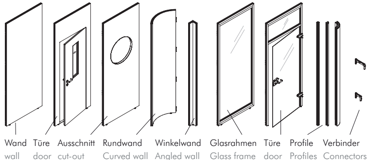
Besprechungskabinen in Leichtbauweise mit Glasfensterausschnitt Meeting cabins in Lightweight construction with glass window cutting
